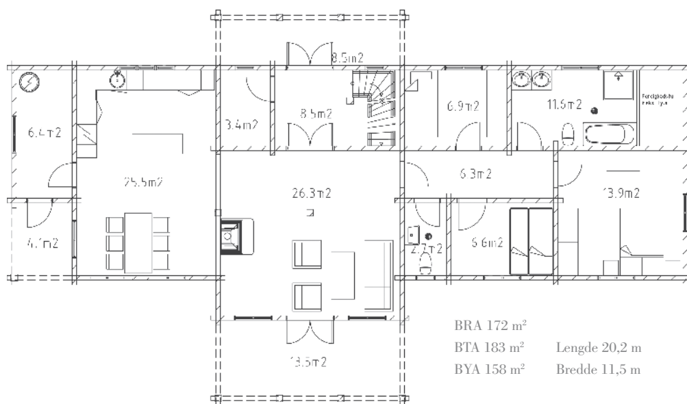
1. etg.
