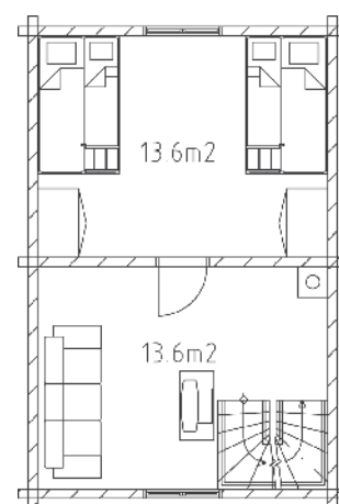
2. etg.
